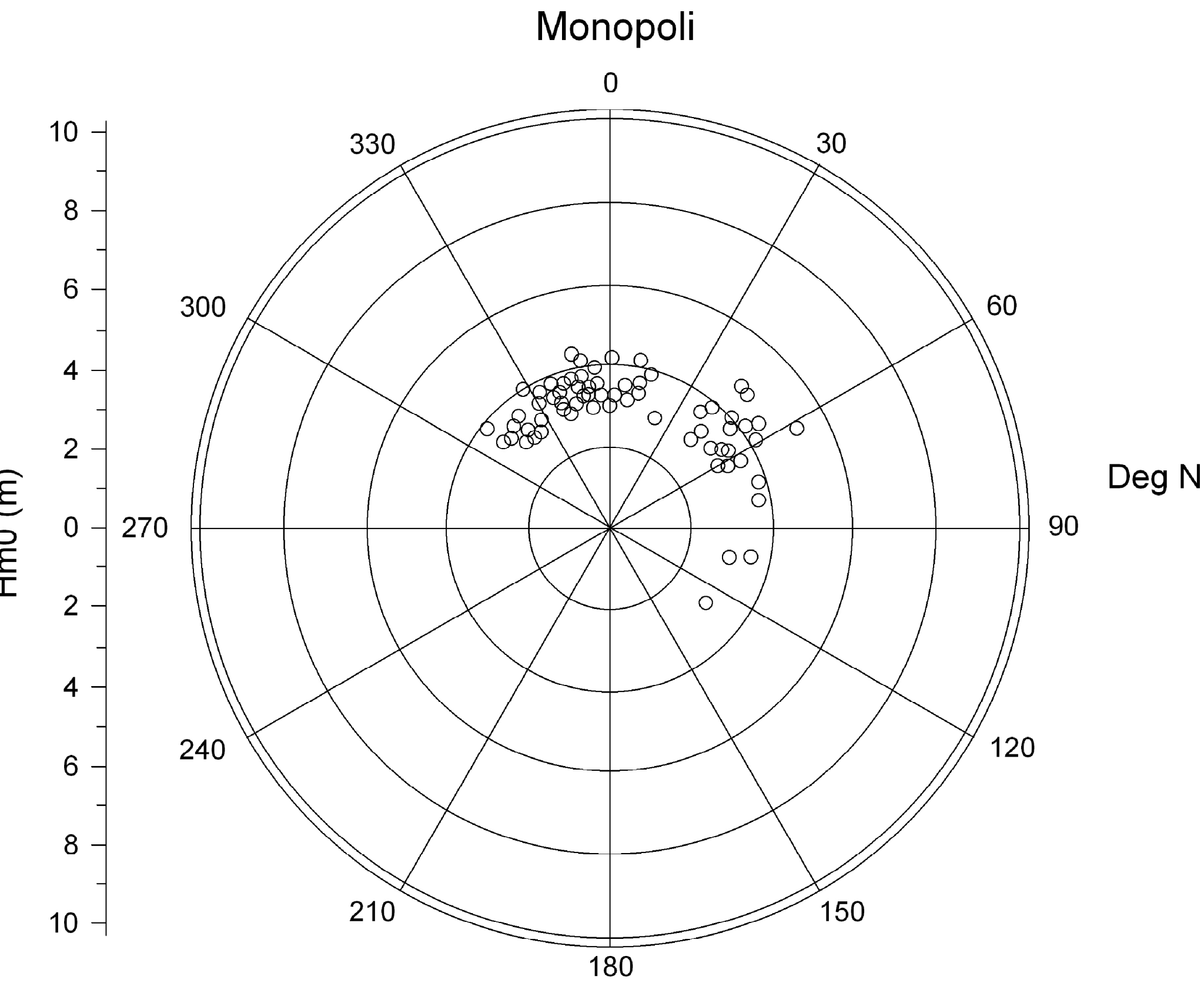
Altezza d'onda massime registrate dalla stazione di Monopoli
